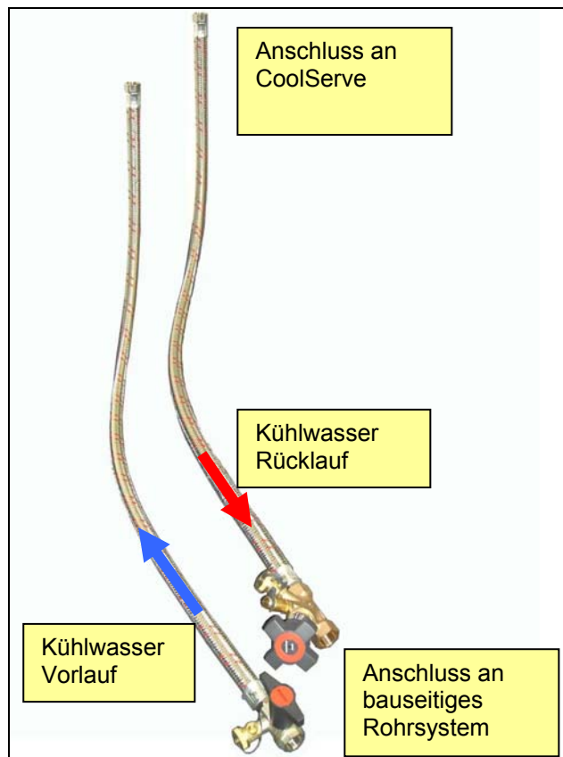
Bild Anschlusset
