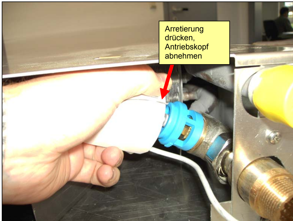
Abbildung Demontage Ventiltrieb durch Drücken der Arretierung
