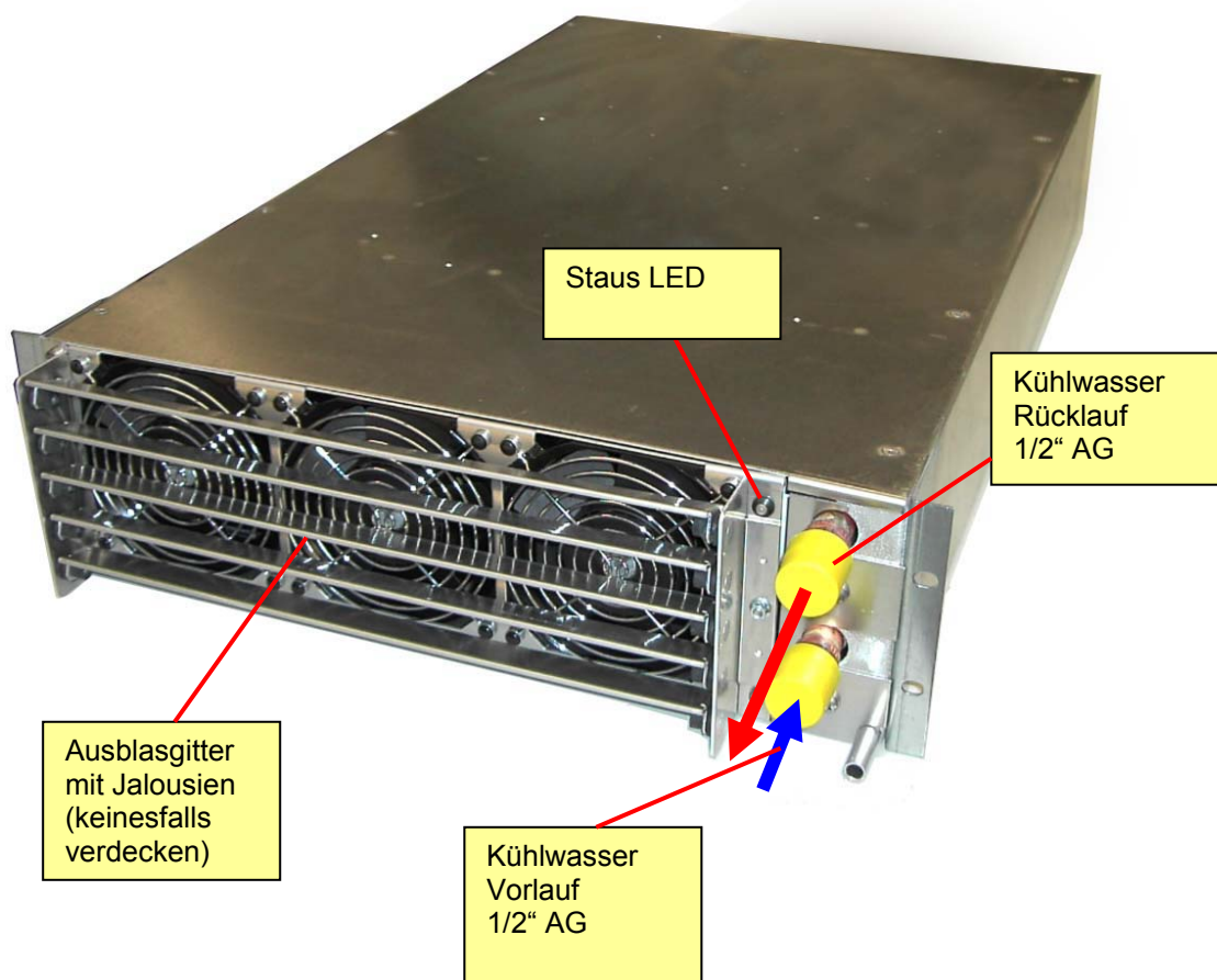
Abbildung CoolServe Frontseite / Anschlüsse
