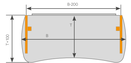
Gestellbreite = B-200mm
