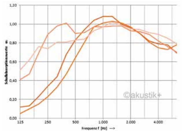
Schallabsorptionswerte für Perforation FINEST (1,8/1,8/0,5mm)
