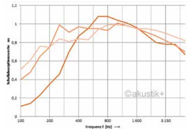
Schallabsorptionswerte für Perforation FINEST (1,8/1,8/0,5mm)
