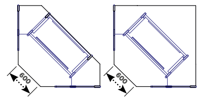
Trapèz. à 90°
